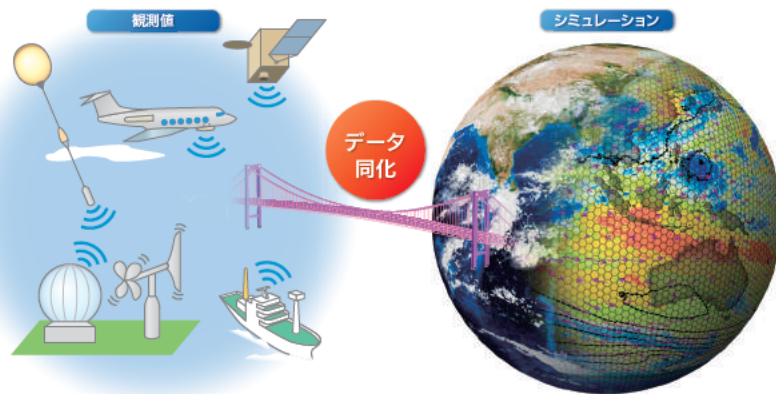
図2 データ同化
