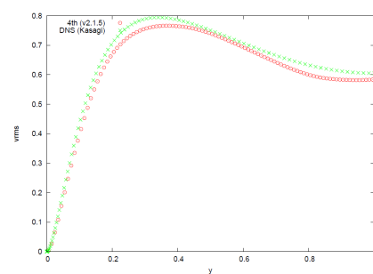
乱流強度 (壁面鉛直方向)
