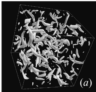
Q = 10 の等値面 ( t = 3.792 ). (a) DNS ([1] より引用) (b) FFV-C (CSM)
