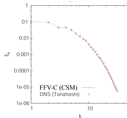
エネルギースペクトル ( t = 3.792 )
