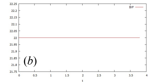
(a) 速度発散値の最大値および (b) 圧力ポアソンの反復回数
